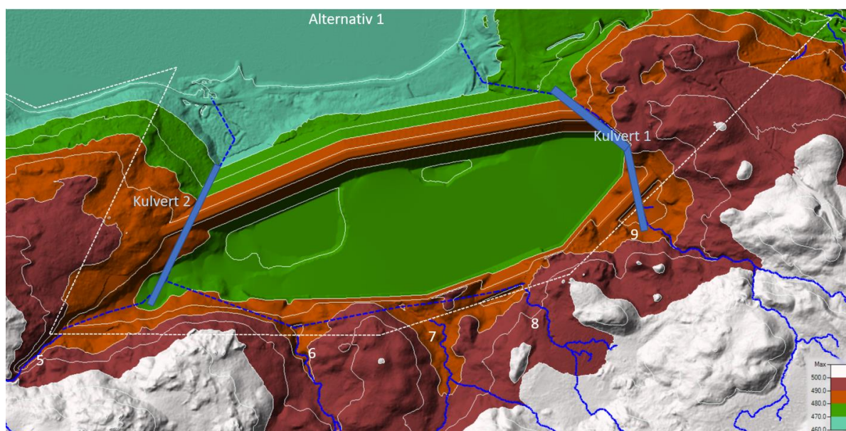
Figur 3-6: Denne løsningen innebærer å føre bekk 9 i kulvert ned til Hudningsvatnet gjennom Kulvert 1. Blå stiplet linje er kanal, mens tykke blå linjer er kulverter.
