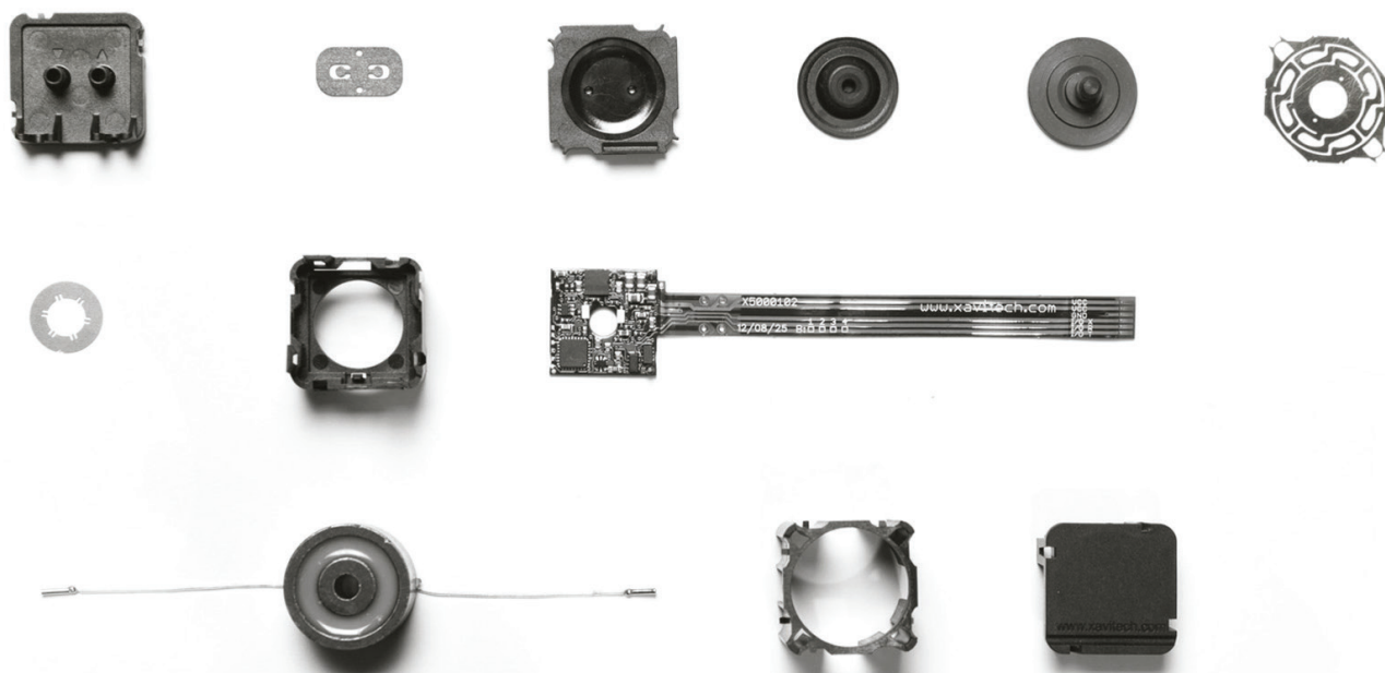
KOMPONENTER TILL EN AV XAVITECHS PUMPMODELLER
