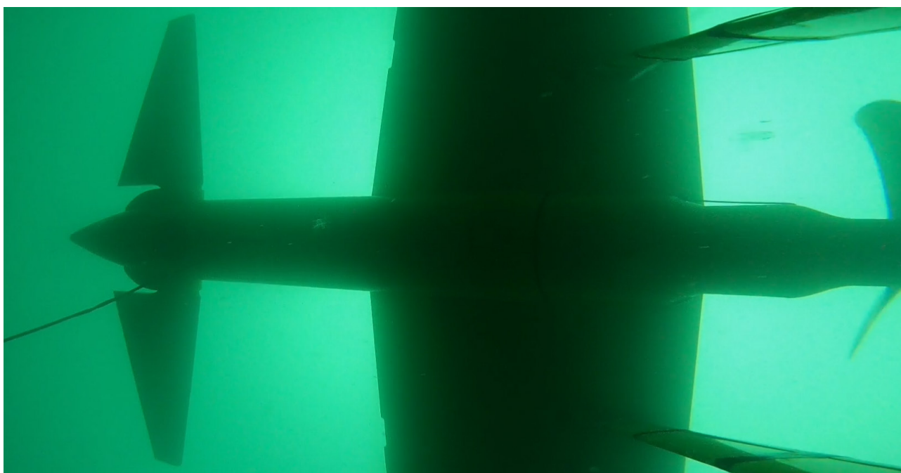
Minestos marina kraftverk DG100 i drift i Vestmannasund, Färöarna under sommaren 2021.
