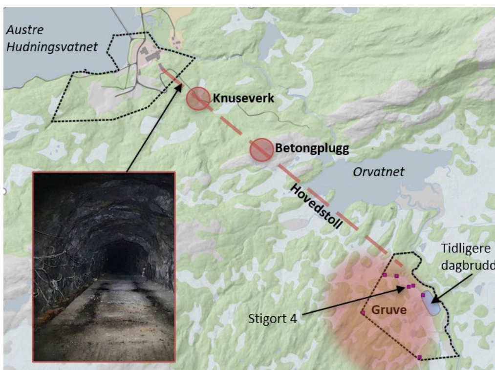
Figur 2-5: Kartet er en illustrasjon som viser prinsipp for forhold under bakken. Rød stiplert linje i kartet viser omtrentlig trasé for hovedstollen som leder frem til gruven under bakken. Gruven er markert som rød oval sirkel. Inne i hovedstollen er det et knuseverk og en betongplugg. Stigort 4 (sjakt 4) er en skråliggende gruvegang som i dag har vannoverløp. Bildet er tatt fra hovedstollen, hvor kanalen med gruvevann kan skimtes på venstre side av veien.
