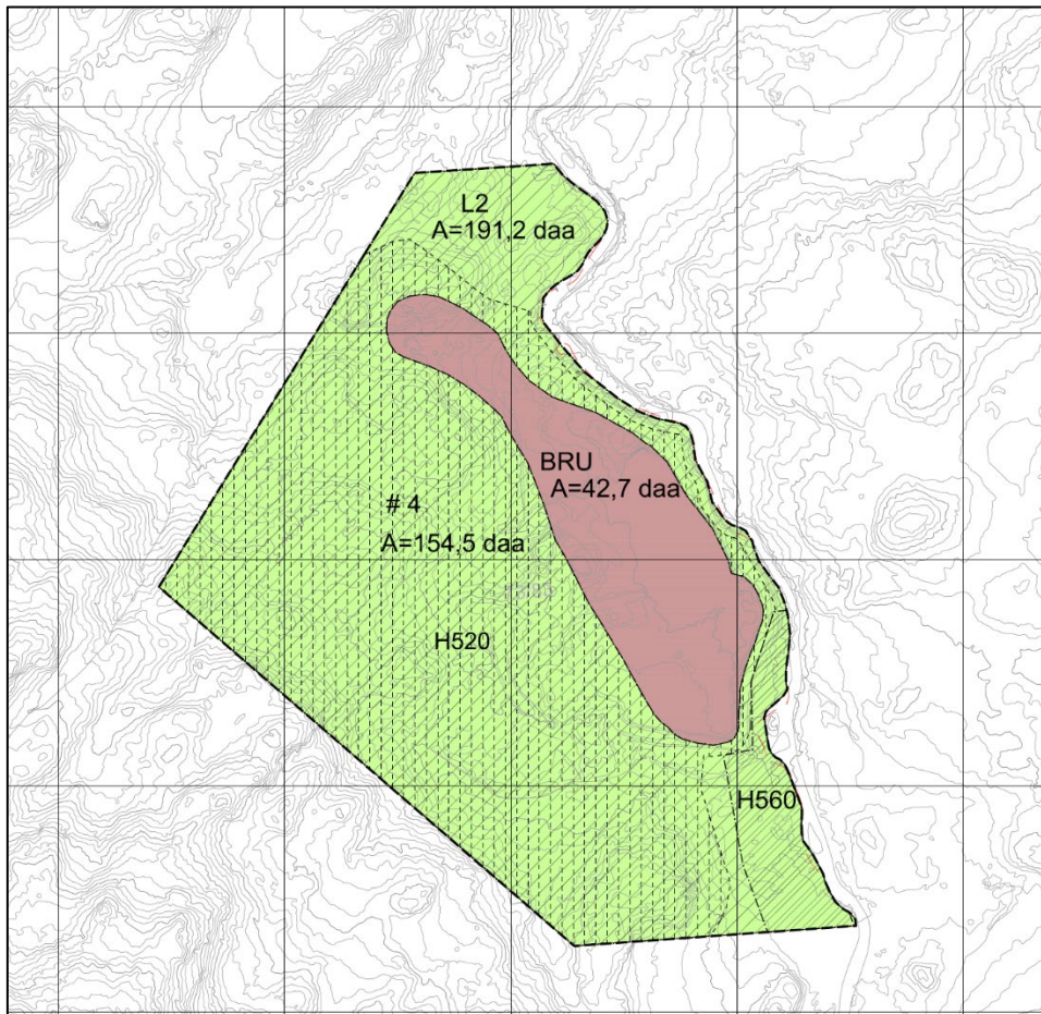
Figur 2-12: Plankartet viser arealdisponeringen ved planområdet sør for Orvatnet, ved tidligere dagbruddsområde. BRU markerer arealet for nytt dagbrudd.
