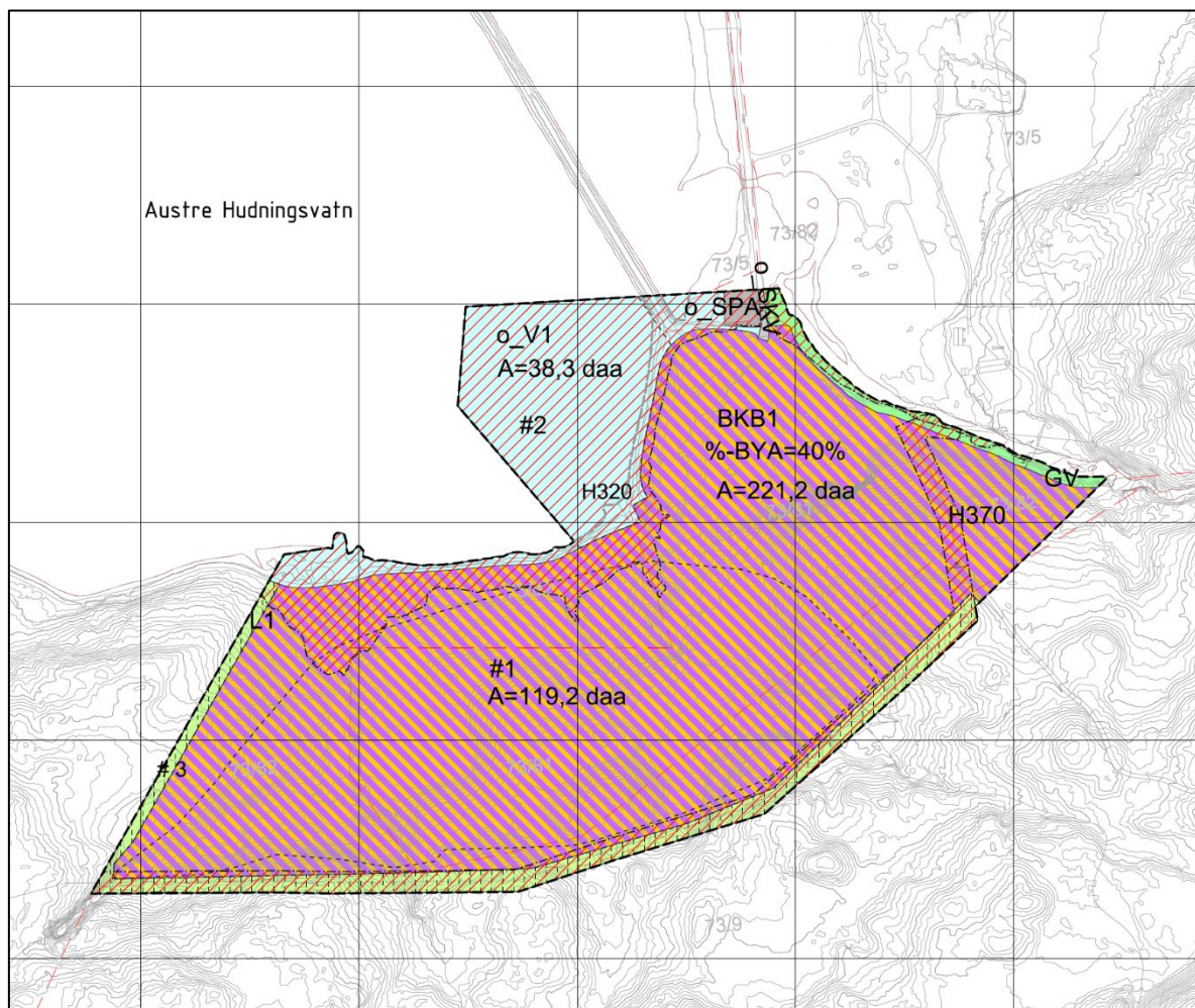
Figur 2-11: Plankartet viser arealdisponeringen ved sør-østlig ende av Austre Hudningsvatnet. Renset vann skal slippes ut i o_V1 (område #2).
