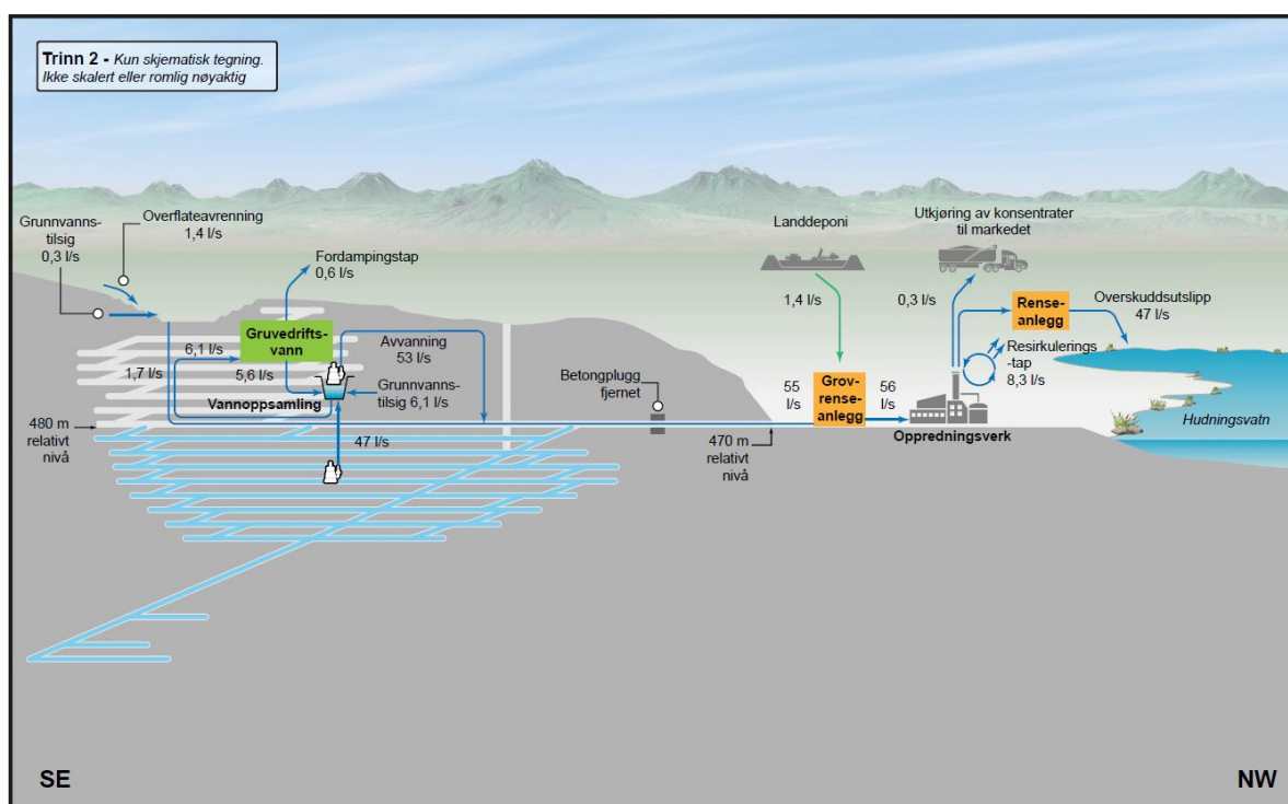
Figur 2-15: Trinn 2: Gruvedriften har startet mens resten av gruva tømmes for vann. Sige vann fra landdeponi og vann fra tømming av gruva brukes i oppredningsprosessen i oppredningsverket. Vann fra gruvetømming som ikke inngår her, ledes til renseanlegg før utslipp til Hudningsvatnet. Kilde: SRK, Vedlegg 5.
